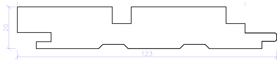
Profile B3
